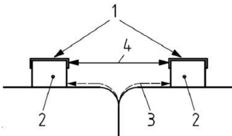
Obr. 2 Povrchová vzdálenost a vzdálenost 1 vodivý povrch 2 připojovací svorka (pack RESS nebo RESS) 3 povrchová vzdálenost 4 vzdálenost
